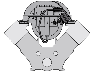
Schaltsaugrohr an einem V-Motor
